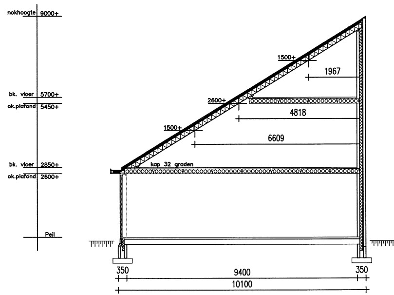
Doorsnedes woning
